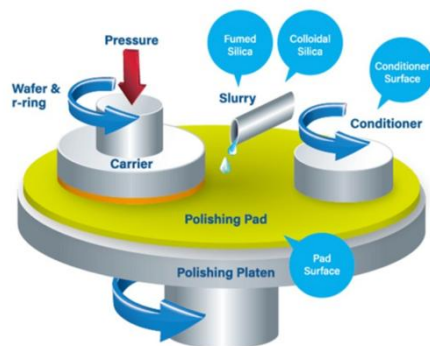
圖 17：CMP 製程
